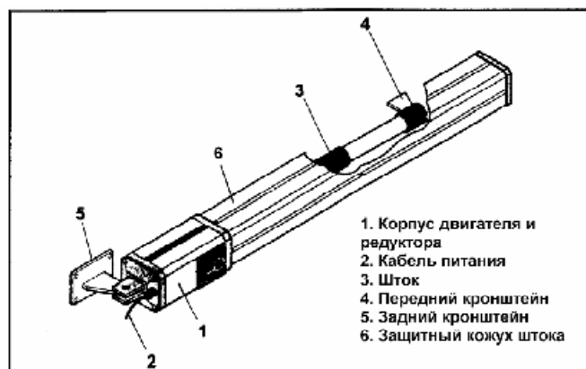
Рис. 1 Состав привода.
