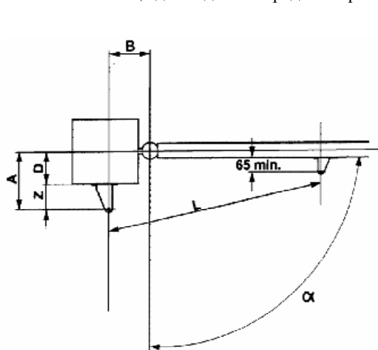
Рис. 5 Основные размеры для установки привода.
